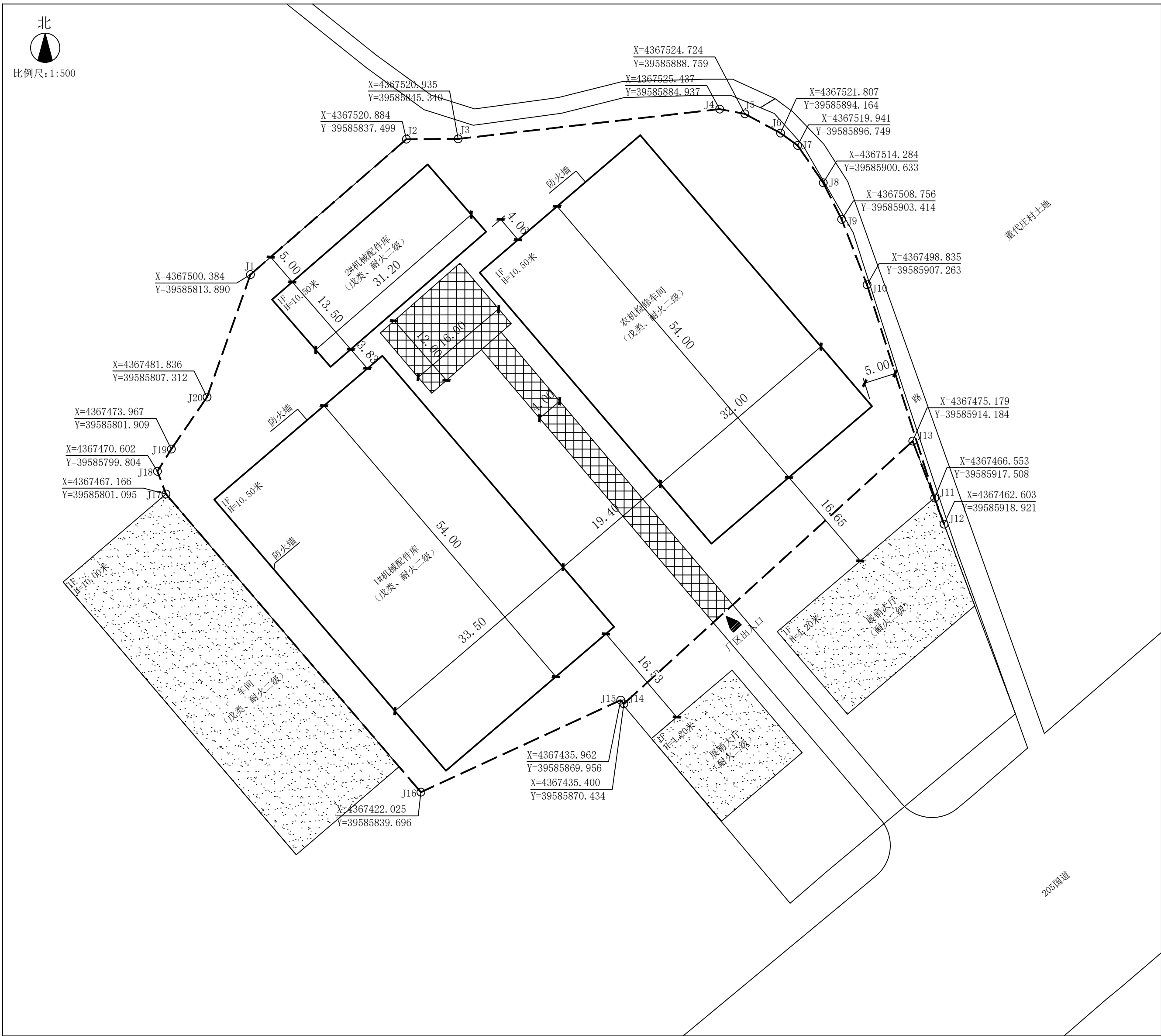
建、构筑物一览表
